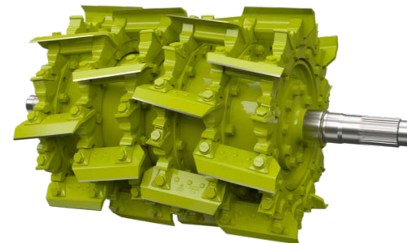
V-FLEX із напівножами для подвоєння довжини подрібнення за симетричної подачі рослинної маси
