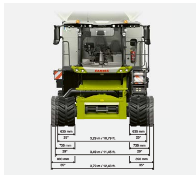
Гусеницы диаметром 635 мм обеспечивают компактность TRION на дороге и повышают его мобильность.
