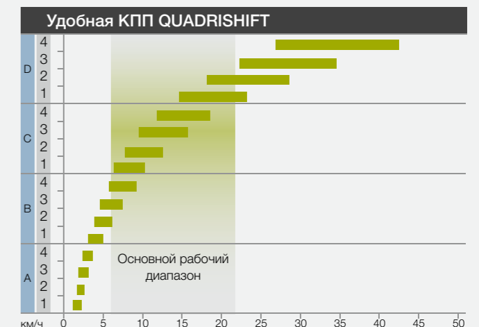
Коробка передач для скорости 40 км/ч при 1400–2200 об/мин Тип шин: 20.8 R 38
