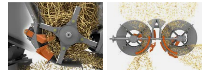
Противорезы и поворотный сегмент днища в измельчителе SPECIAL CUT
